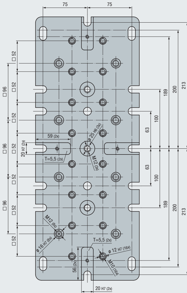
Anschraubbild für Maschinentisch / EvoPoint (Unterseite) Assembly picture for machine table / EvoPoint (bottom)
