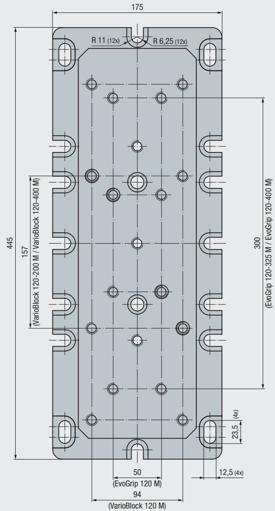
Anschraubbild für EvoGrip / VarioBlock (Oberseite) Assembly picture for EvoGrip / VarioBlock (top)
