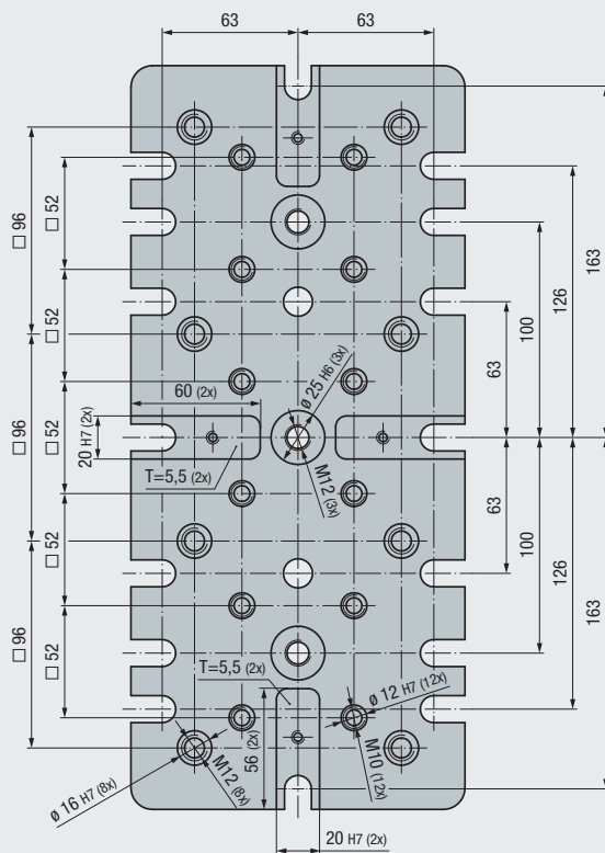
Anschraubbild für Maschinentisch / EvoPoint (Unterseite) Assembly picture for machine table / EvoPoint (bottom)
