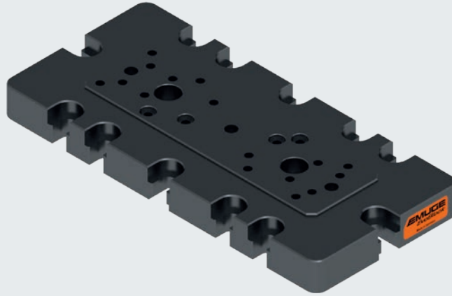
Anschraubbild für Maschinentisch / EvoPoint (Unterseite) Assembly picture for machine table / EvoPoint (bottom)
